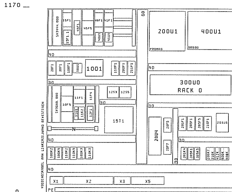
Montageplaat 1150
