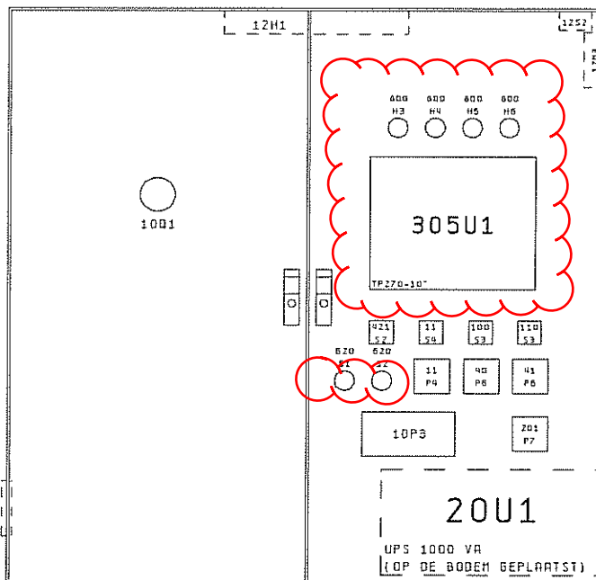
Voor-aanzicht 1200
