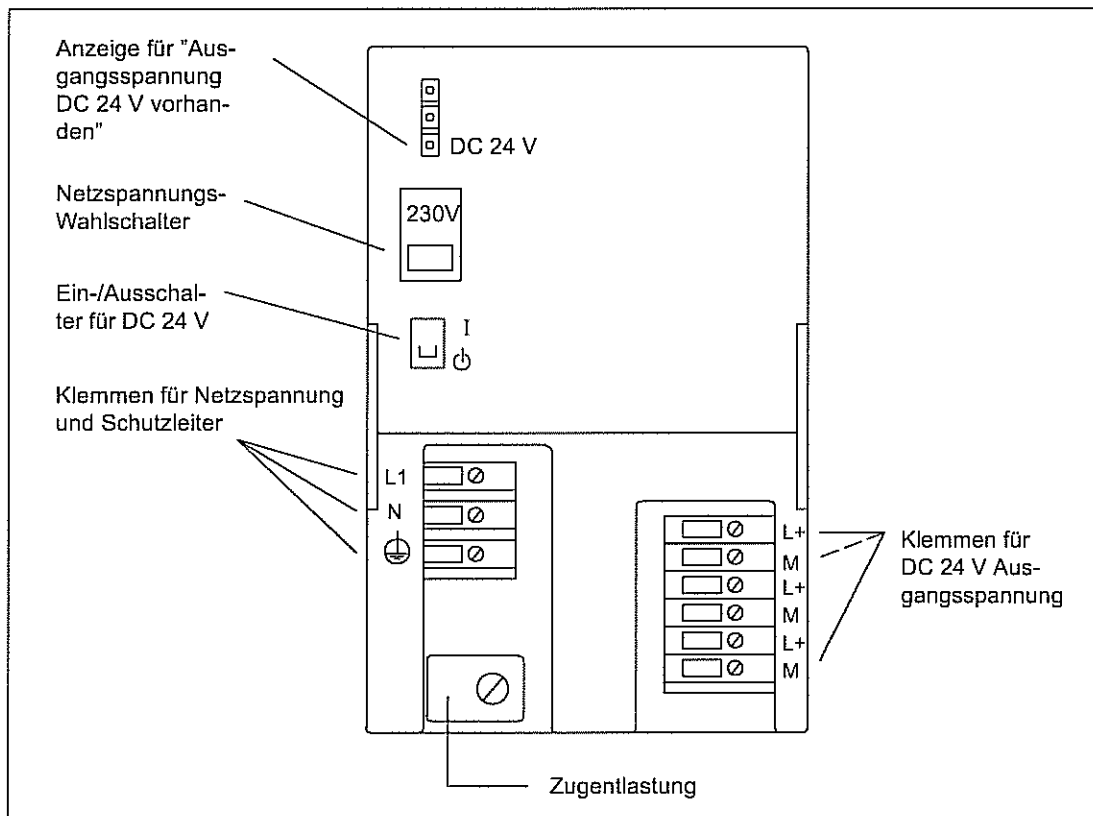
Bild 2-5 Anschlußbild der Stromversorgungsbaugruppe PS 307; 5 A
