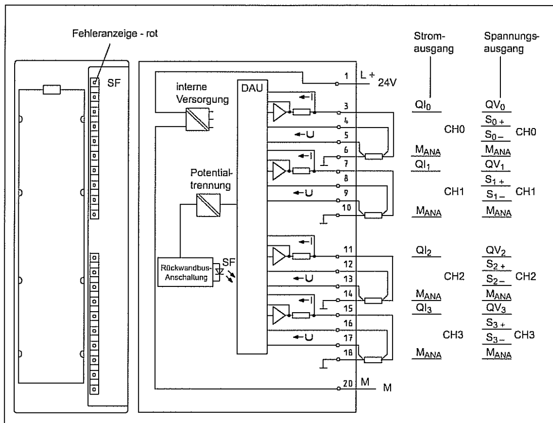
Bild 4-53 Baugruppenansicht und Prinzipschaltbild der SM 332; AO 4 × 12 Bit
