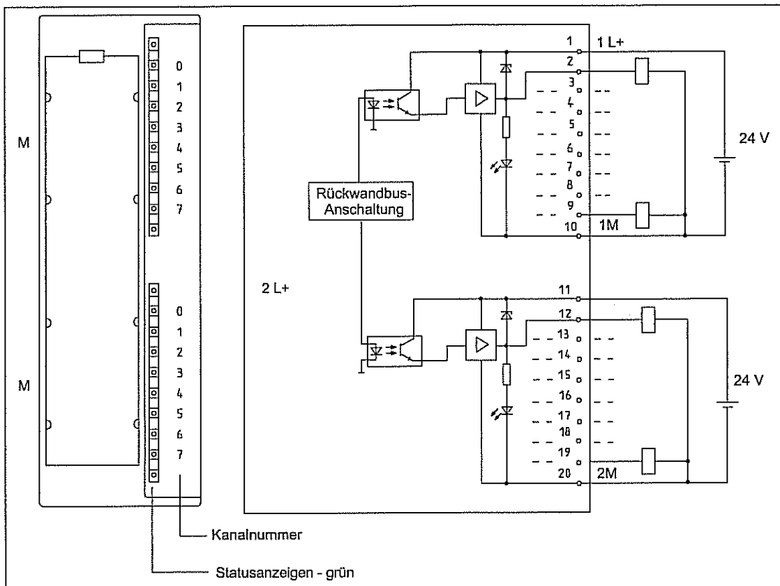
Bild 3-20 Baugruppenansicht und Prinzipschaltbild der SM 322; DO 16 x DC 24 V/0,5 A
