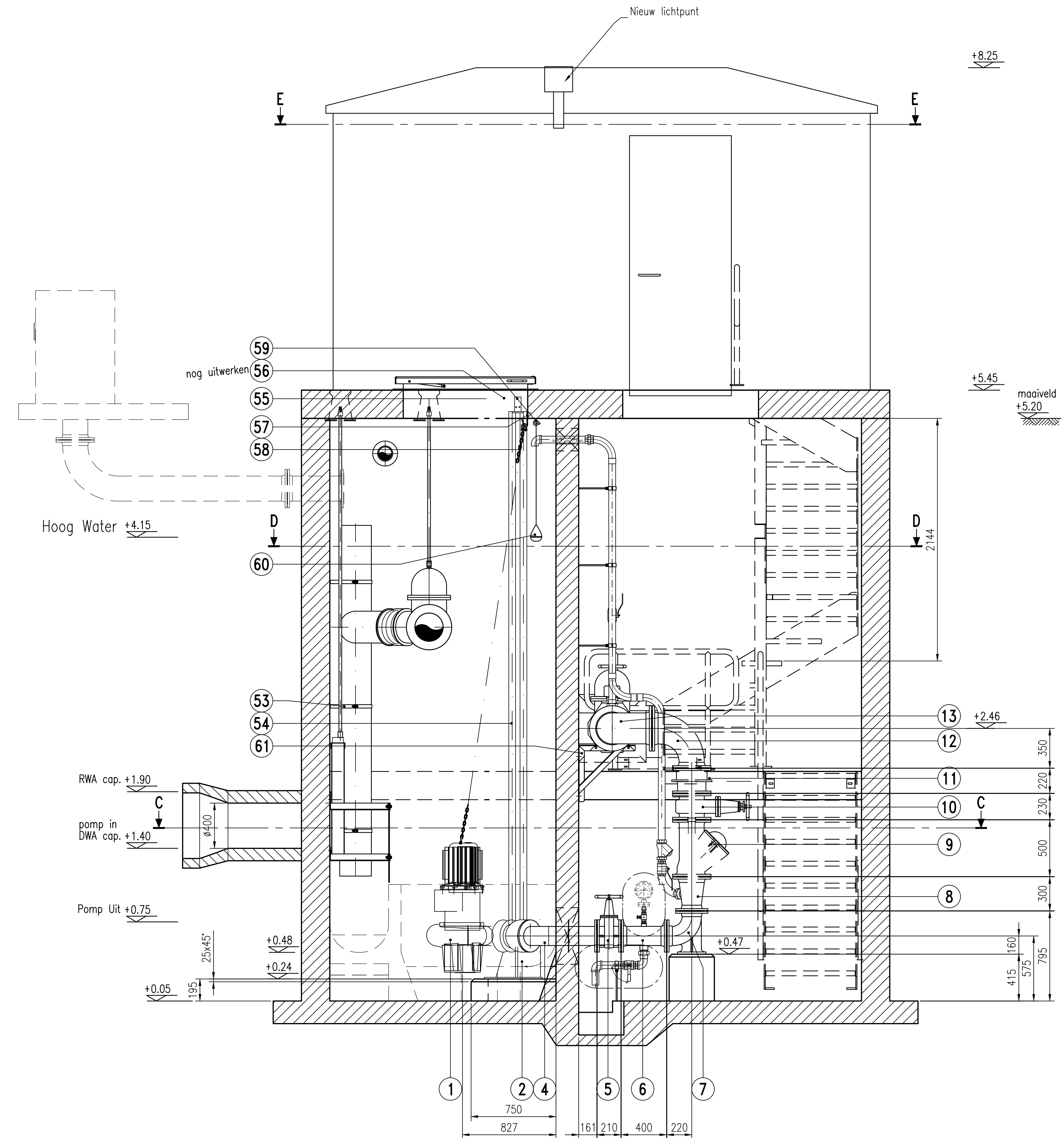
doorsnede A-A
