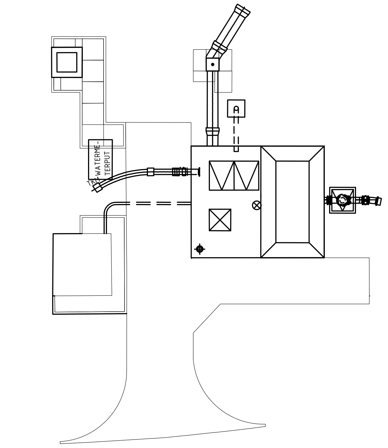
situatie (schaal 1:100)
