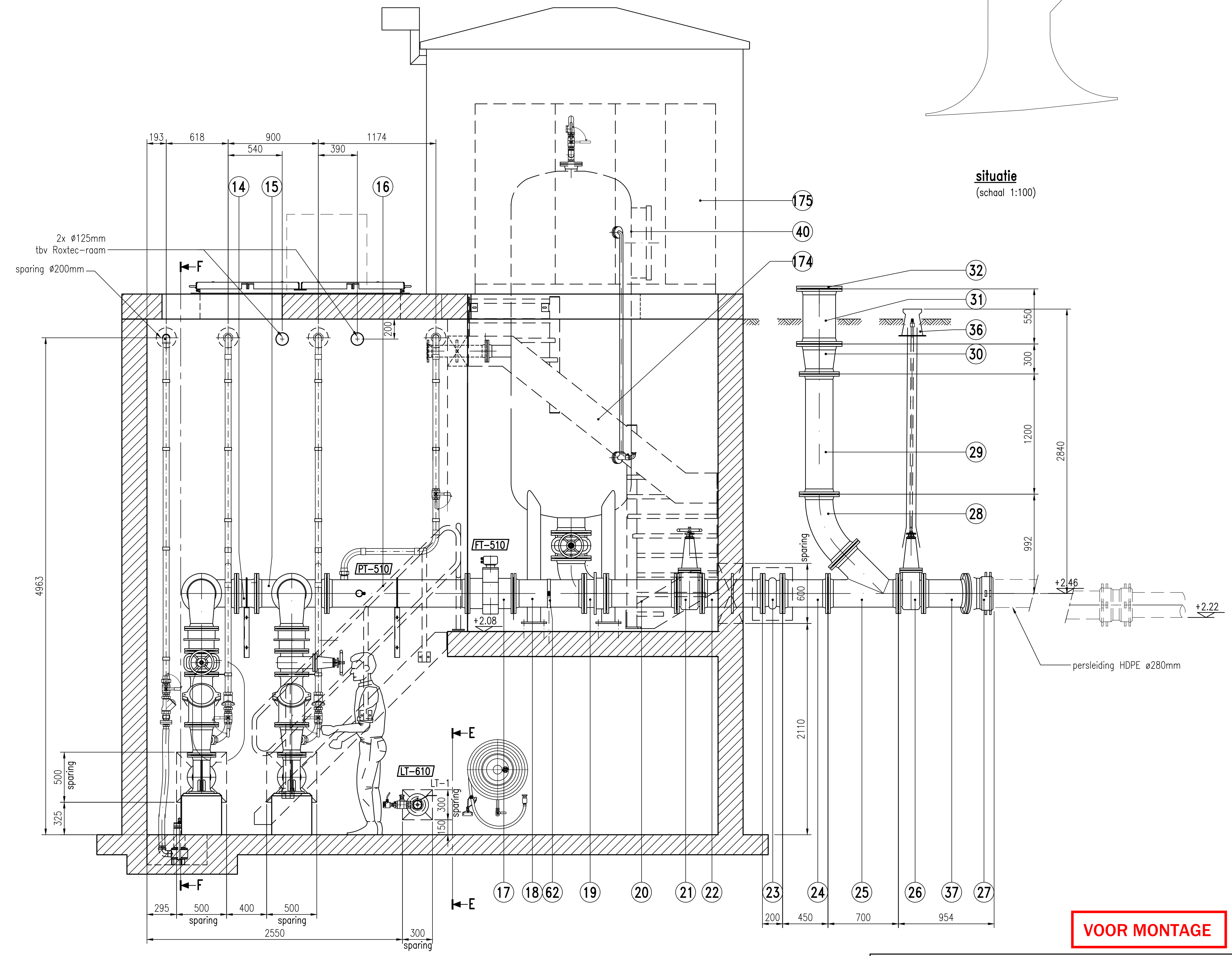
doorsnede B-B
