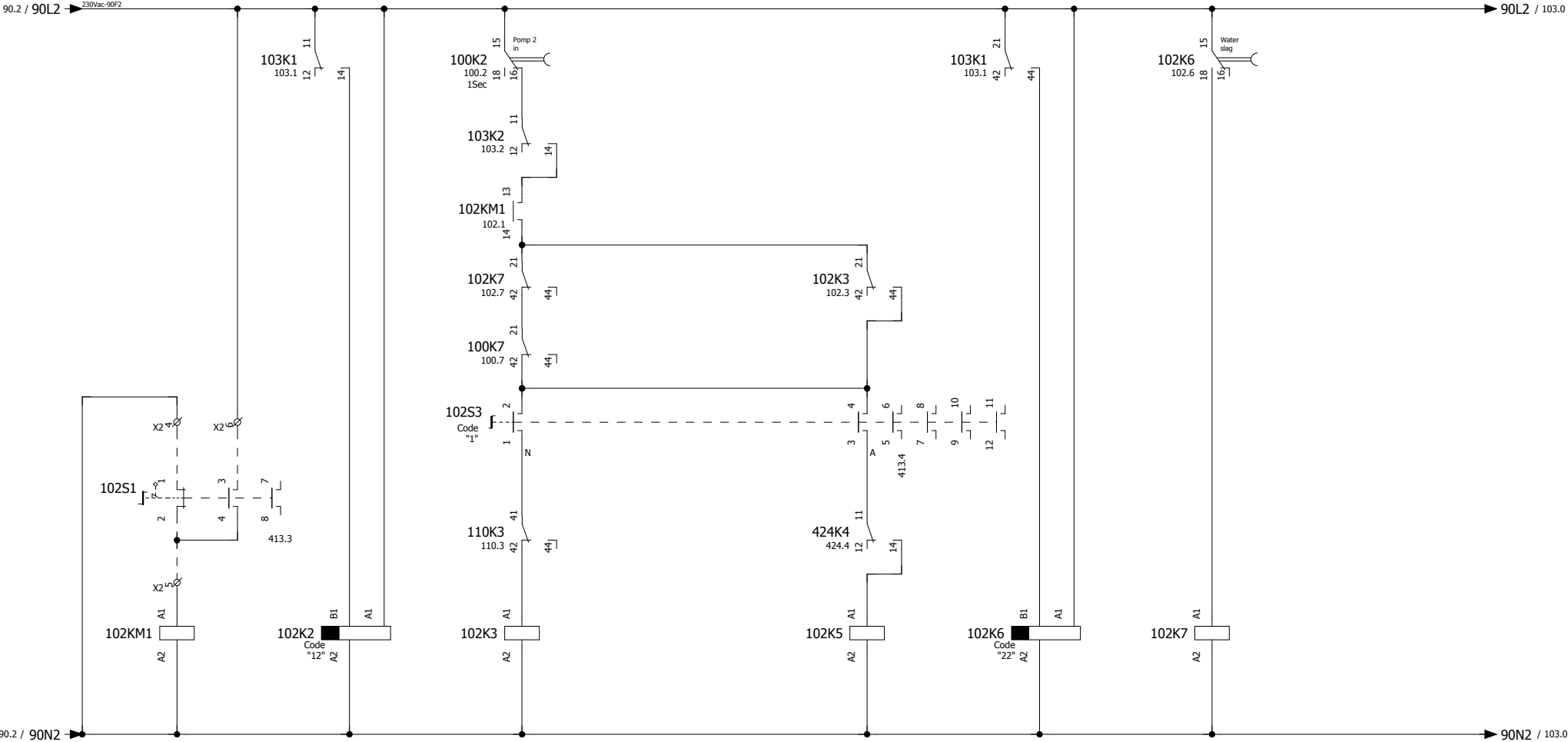
Werschakelaar pomp 2
