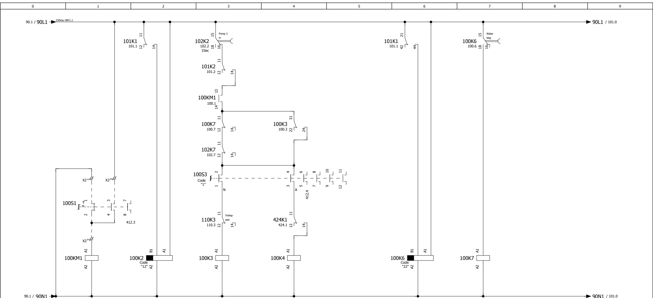
Werkshakelaar pomp 1
